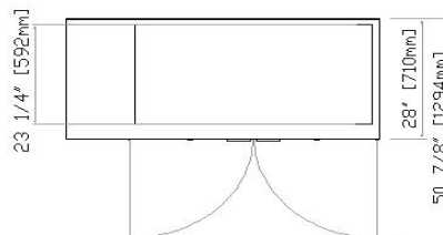
EBB(G)58 TOP
